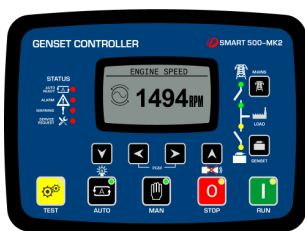
Datakom SMART 500
